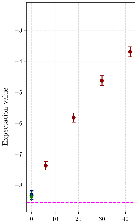
XY ansatz ric-4
