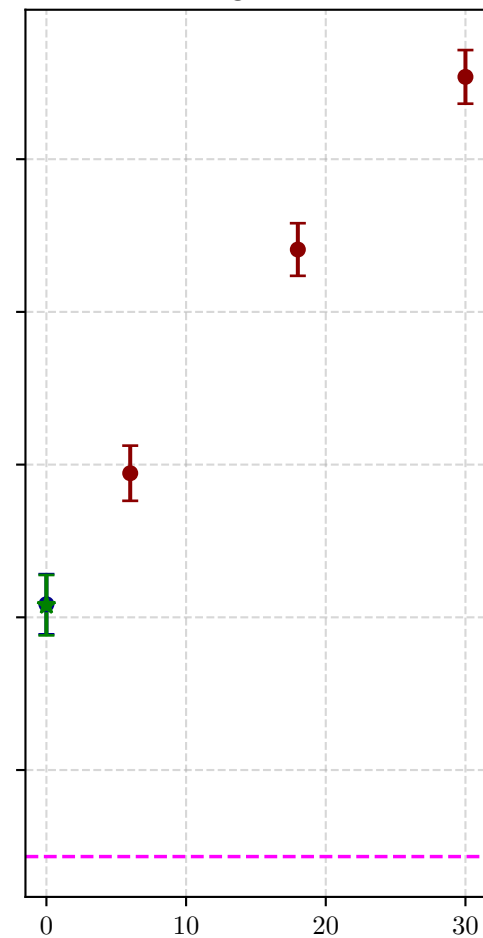
Heisenberg ansatz ric-3
