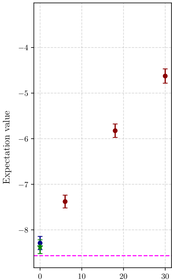
XY ansatz ric-3
