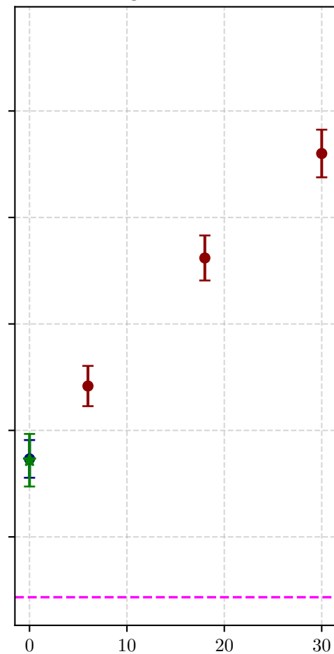
Ising ansatz ric-3
