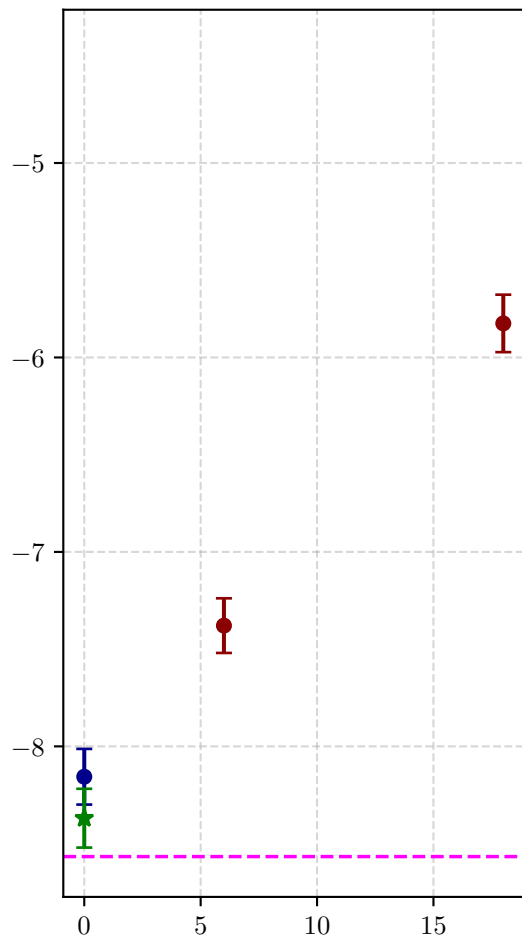
XY ansatz ric-2
